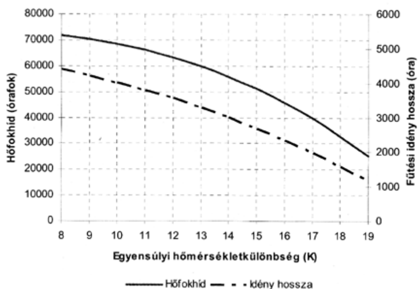
1. ábra: Hőfokhíd és fűtési időny hossza 20 °C belső hőmérséklet esetén az egyensúlyi hőmérséklet-különbség függvényében
